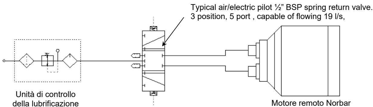
FIGURA 8 – Esempio di sistema di controllo dell'avvitatore
