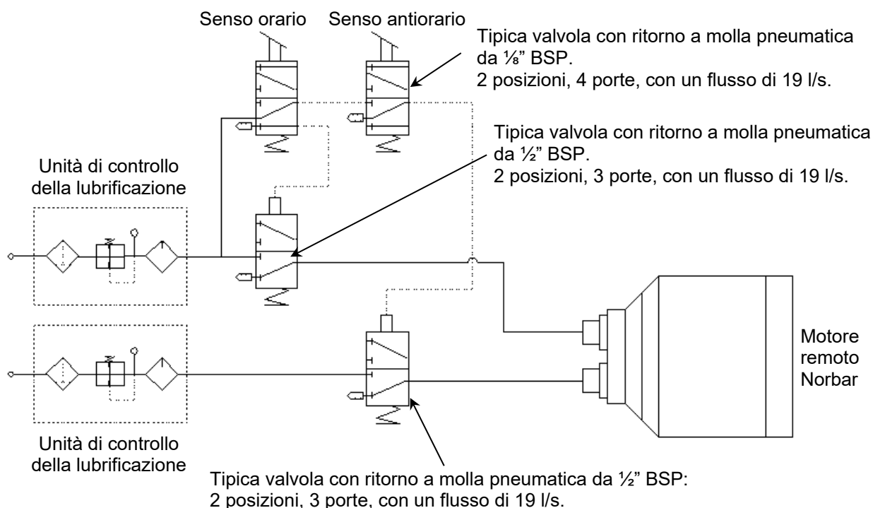
FIGURA 7 – Esempio di sistema di controllo dell'avvitatore
